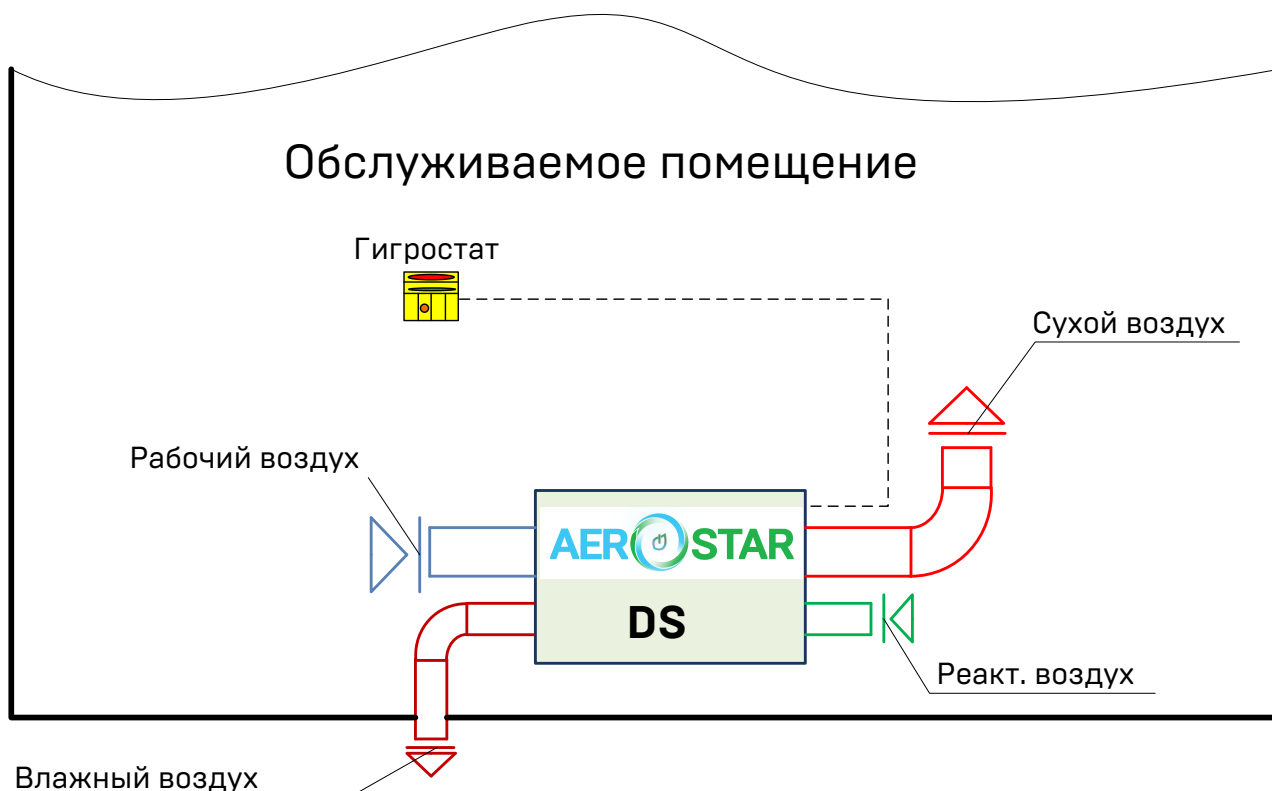
Рисунок 4.7 – Работа осушителя в режиме "сушка" (внутреннее исполнение)
