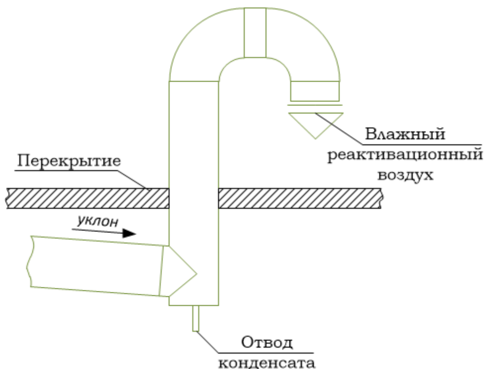
Рисунок 4.9 – Пример прокладки вертикального воздуховода выбросного реактивационного воздуха
