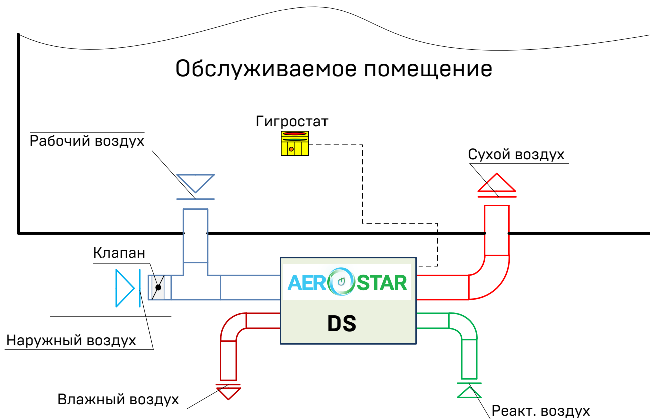
Рисунок 4.6 – Работа осушителя по «закрытой» схеме с подмесом свежего воздуха (наружное исполнение)
