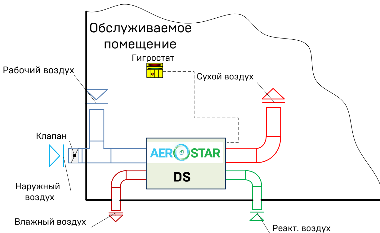
Рисунок 4.5 – Работа осушителя по «закрытой» схеме с подмесом свежего воздуха (внутреннее исполнение)
