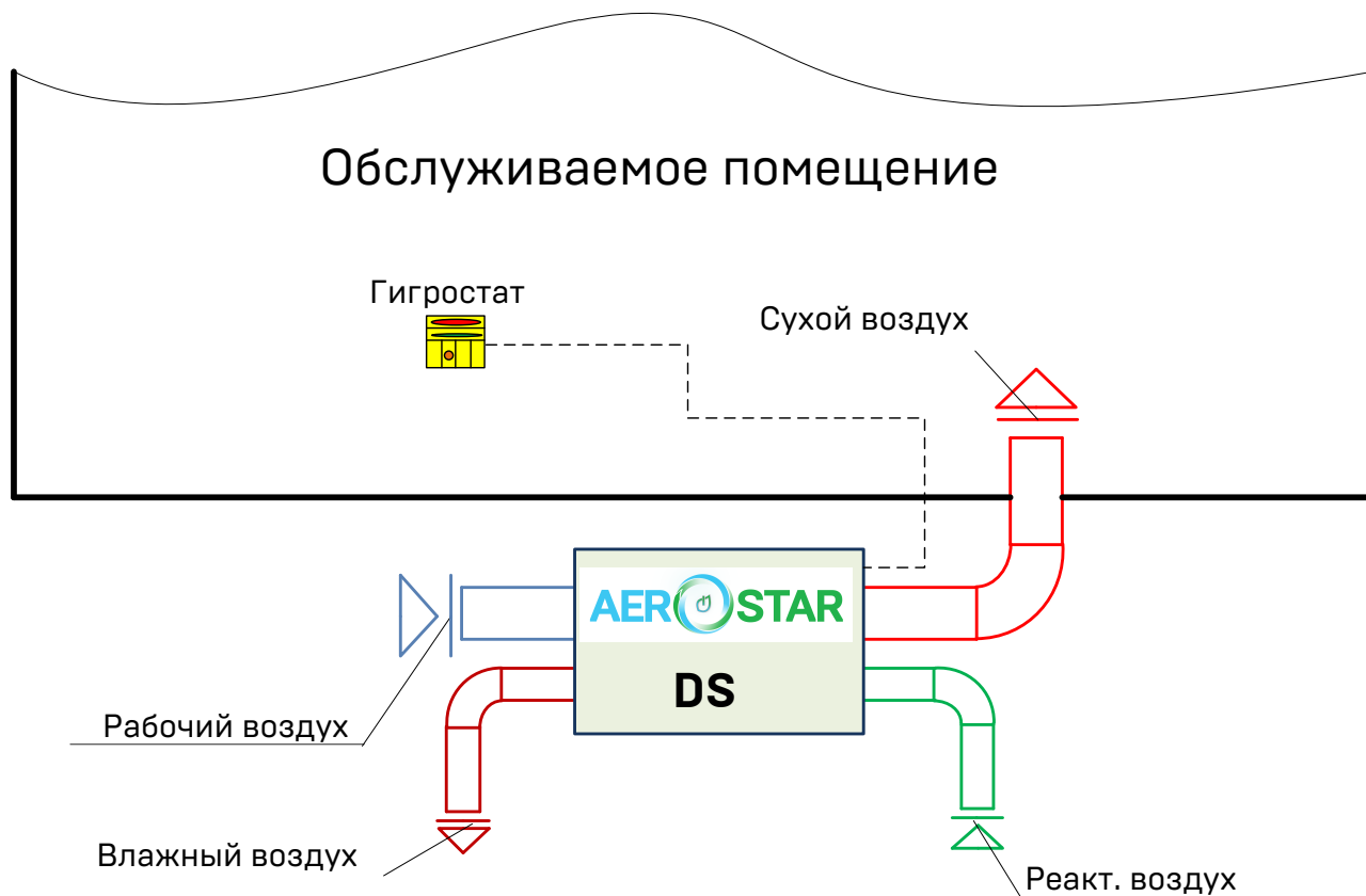
Рисунок 4.4 – Работа осушителя по «открытой» схеме (наружное исполнение)
